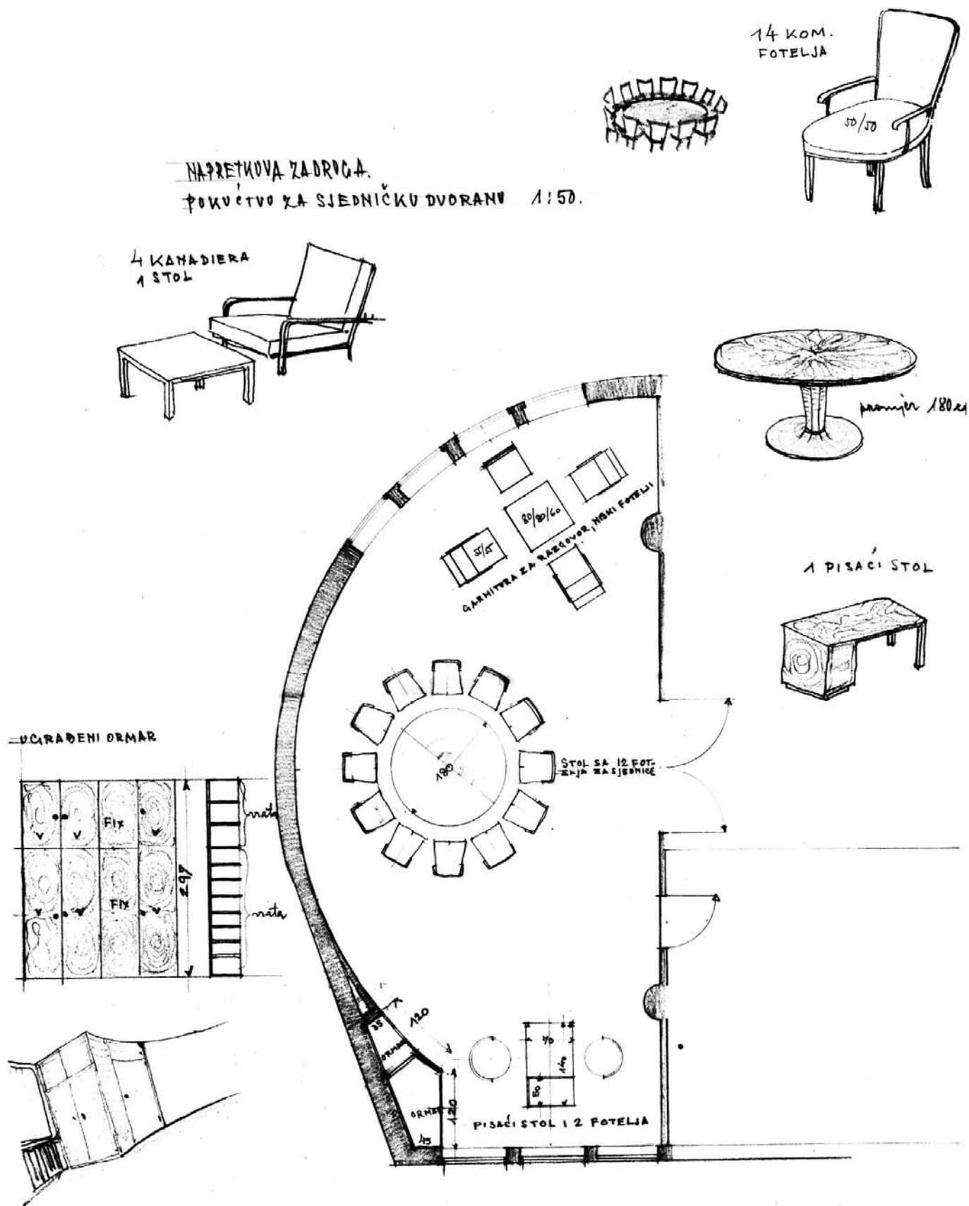
Stambeno-poslovna zgrada "Napretkova zadruga", skica interijera / The "Napretkova zadruga" housing and business building, study for the interior, Zagreb, Bogovićeva 1, 1936-37.
