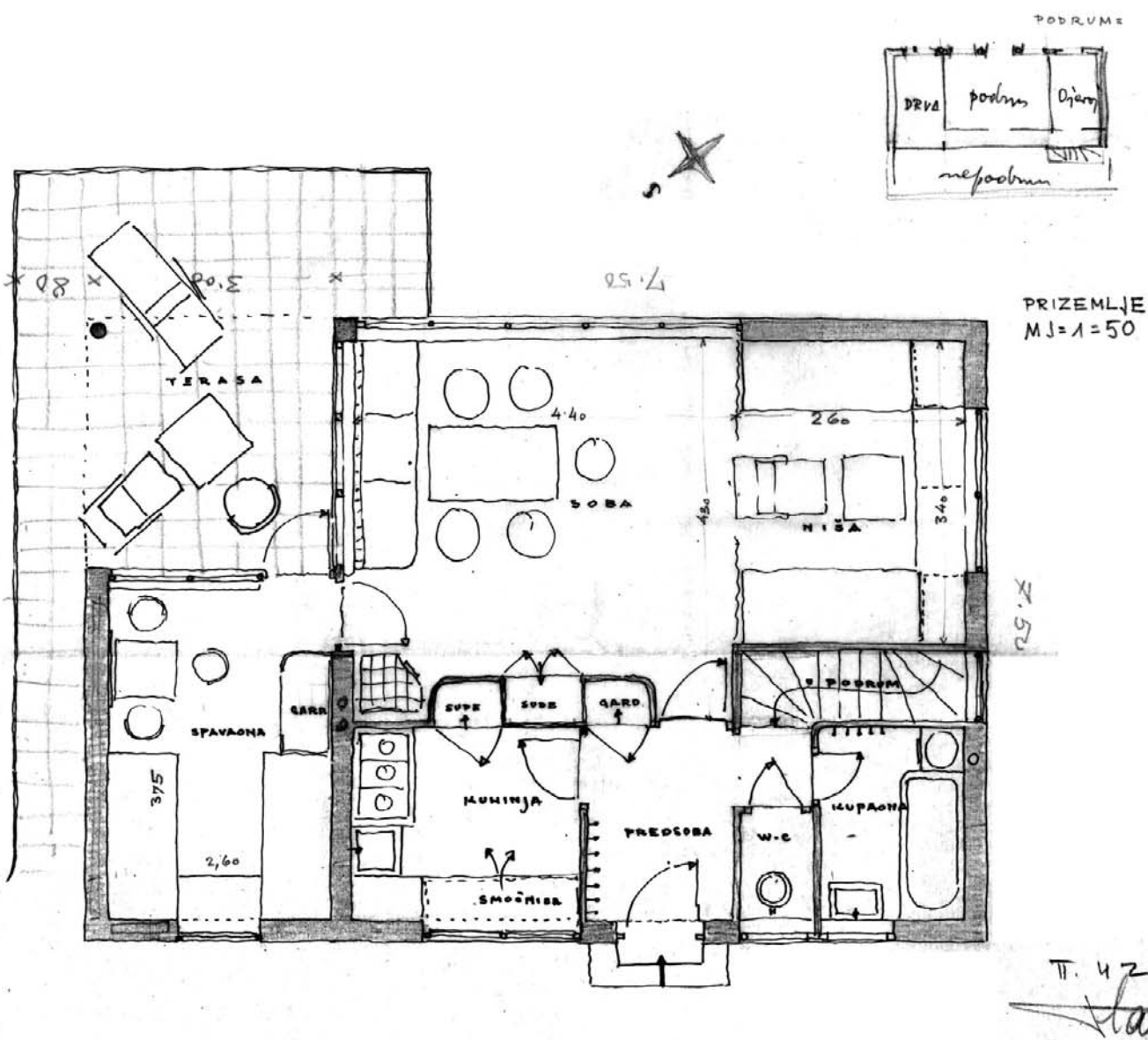
Obiteljska kuća Frković s gospodarstvom, idejni nacrt / The Frković farmstead, Samobor, project, Lešće 15, 1941-44.
