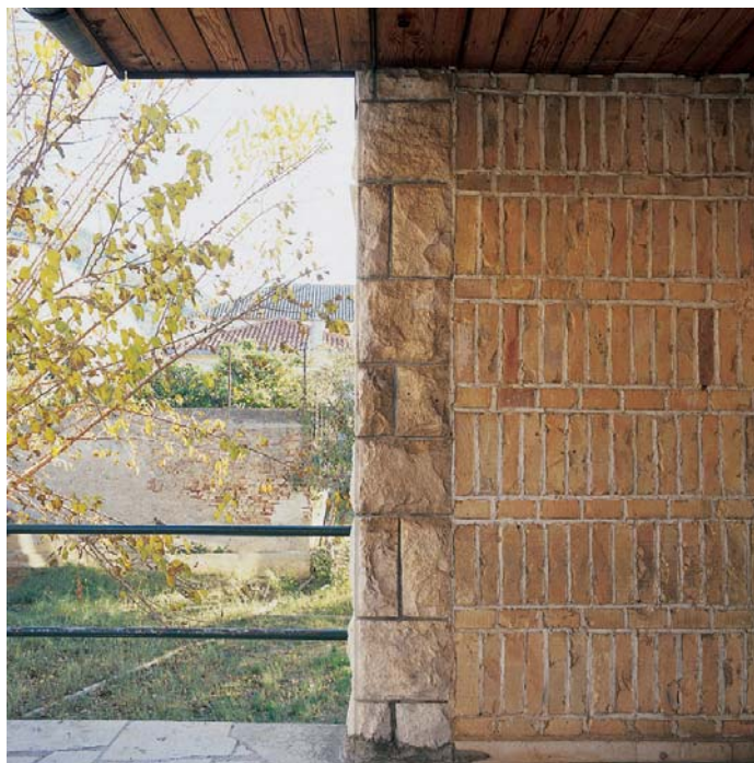
Dječji centar / The Daycare Centre , Komiža, 1964. (foto: Damir Fabijanić)
